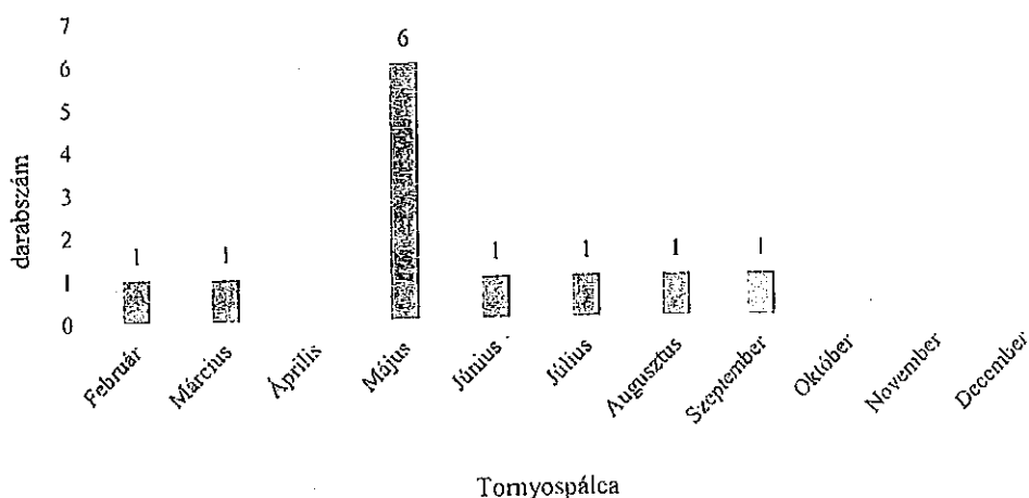
Csőtörések kimutatása 2018.
